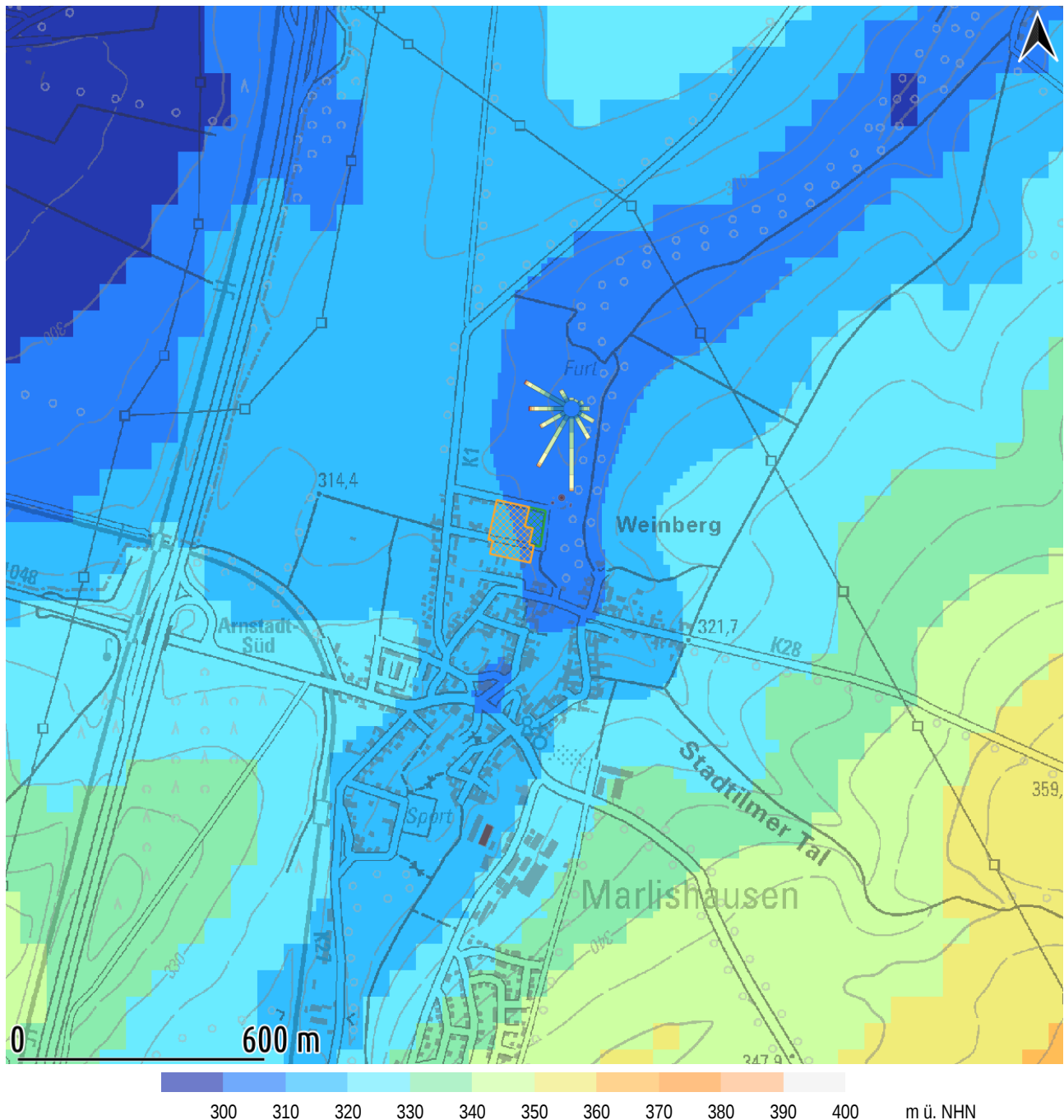
Abb. 5: digitales Höhenmodell | Auszug 2560 x 2560 m 2 von {32640832;5631088} bis {32643392;5633648} | Kartenhintergrund: DTK25, TLBG
