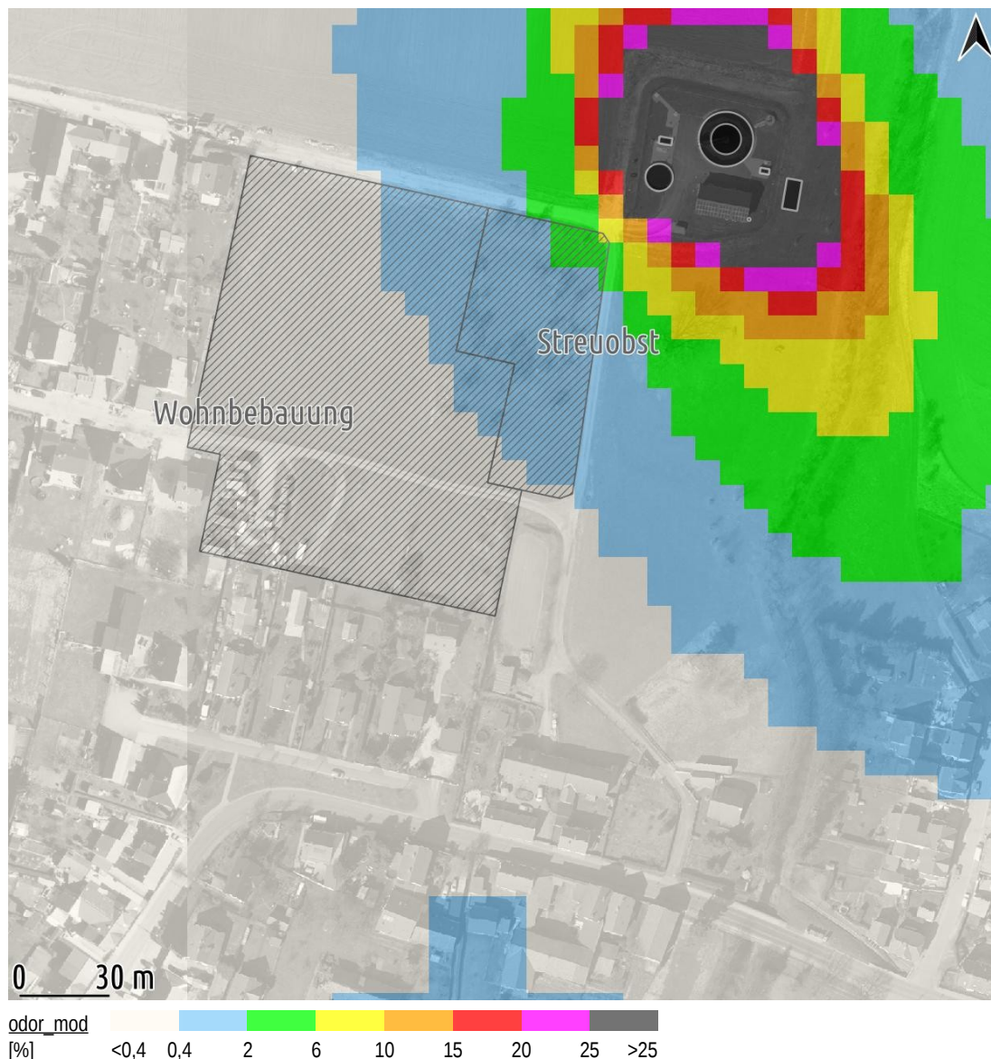
Abb. 9: belästigungsrelevante Geruchsstundenhäufigkeiten im Bereich 328 x 328 m 2 von {32641941;5632173} bis {32642269;5632501} | Kartengrundlage: DOP20, TLBG
