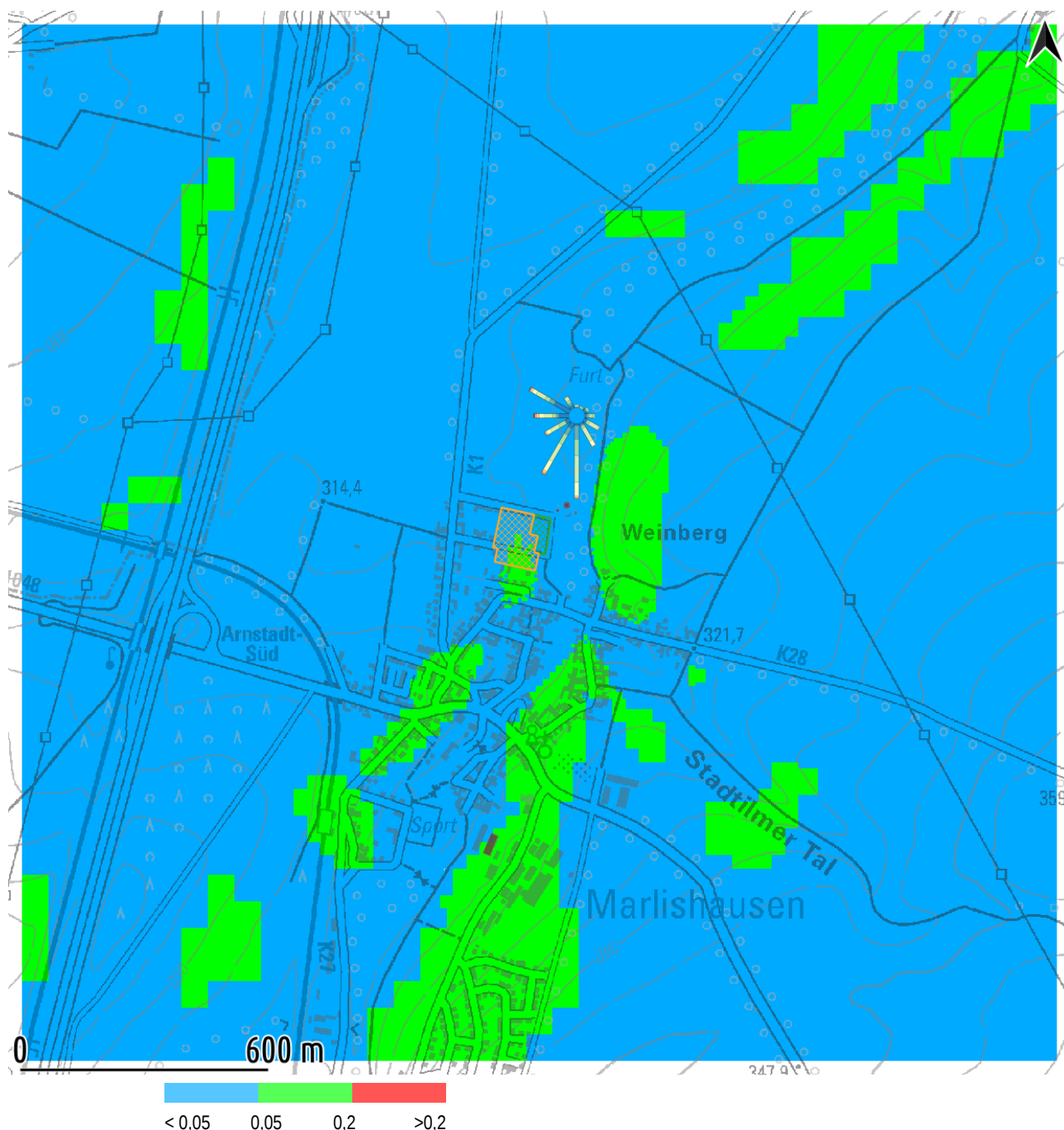
Abb. 6: Geländesteilheit im digitalen Höhenmodell | Auszug 2560 x 2560 m 2 von {32640832;5631088} bis {32643392;5633648} | Kartenhintergrund: DTK25, TLBG
