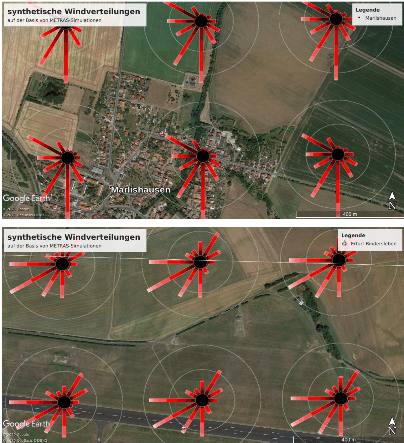
Abb. 8: synthetische Windverteilungen auf der Basis von METRAS-Simulationen (rosa-rot-braun-Balkendiagramme mit schwarzem Zentrum) gemäß [Lit. 19] im Bereich der Emissionsquellen in Marlishausen (Zielbereich) sowie im Bereich der Station Erfurt-Weimar des DWD | Auszug aus GoogleEarth
