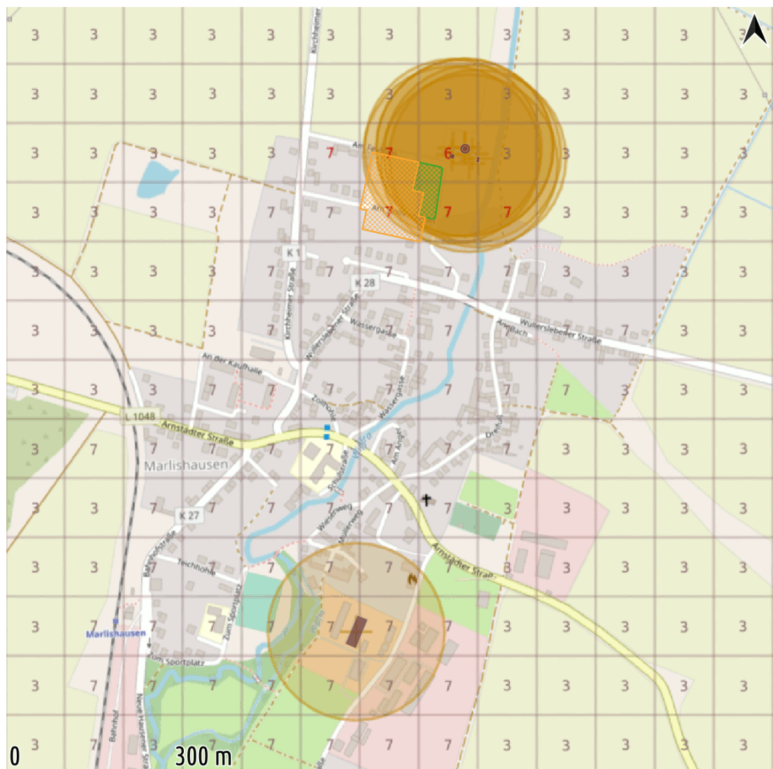
Abb. 7: Rauigkeitsklassen, angepasst für die vorhandene bzw. geplante Bebauung und den entsprechenden Bewuchs, OSM-Auszug 1300 x 1300 m 2 von {32641500;5631400} bis {32642800;5632700} mit der Position des Reit- und Pensionsstalls in der Alten Hausener Straße | Die roten Ziffern kennzeichnen Änderungen gegenüber dem Standard-Kataster. | Kartengrundlage: OpenStreetmap
