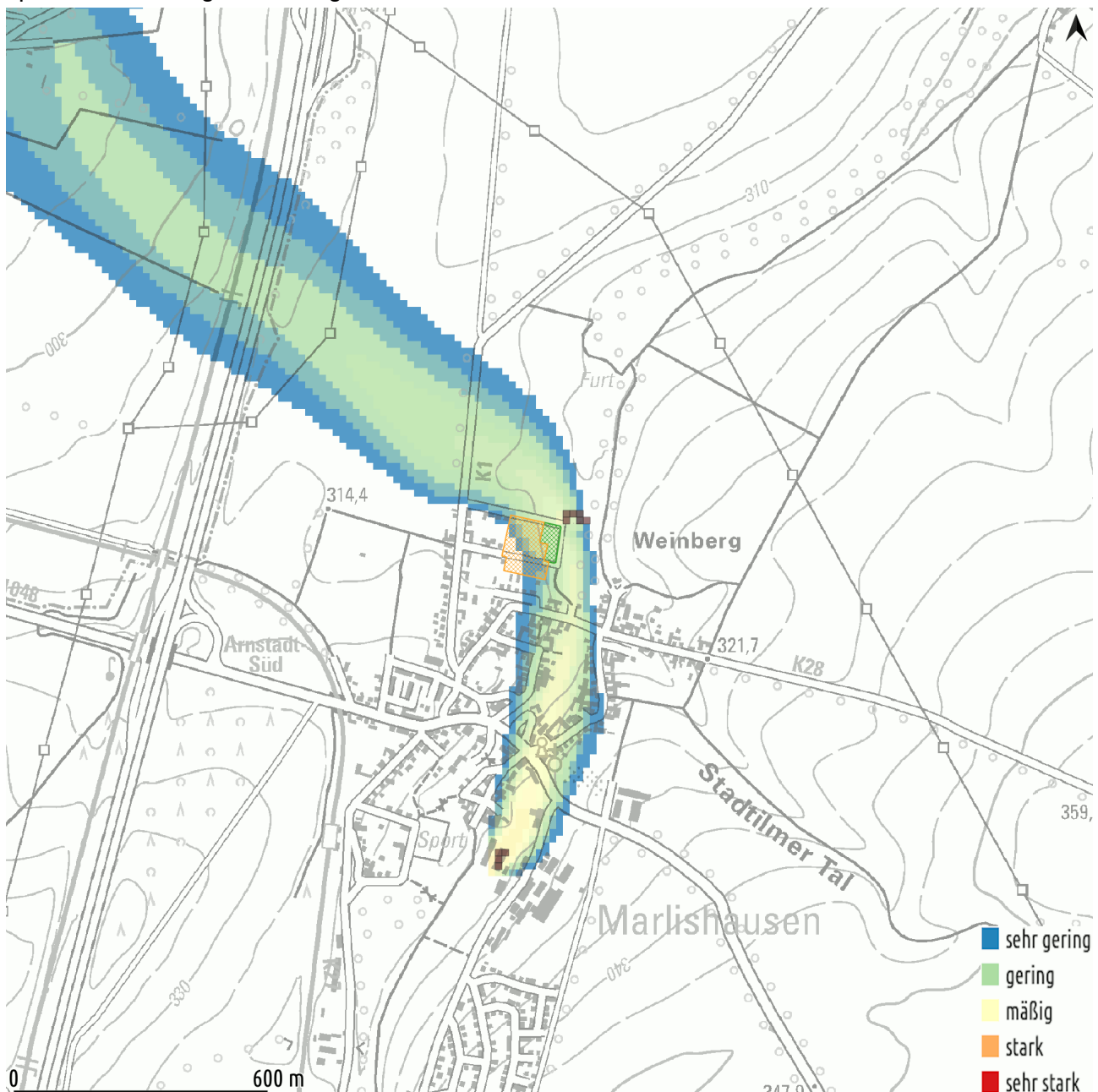
Abb. 8: Intensität bei Ausbreitung von Luftbeimengungen innerhalb der Kaltluft für den Zeitpunkt 3 Stunden nach Eintreten eines entsprechenden Ereignisses | Auszug 2560 x 2560 m 2 von {32640832;5631088} bis {32643392;5633648} mit den aufgerasterten Emissionsquellen | Kartengrundlage: DTK25, TLBG
