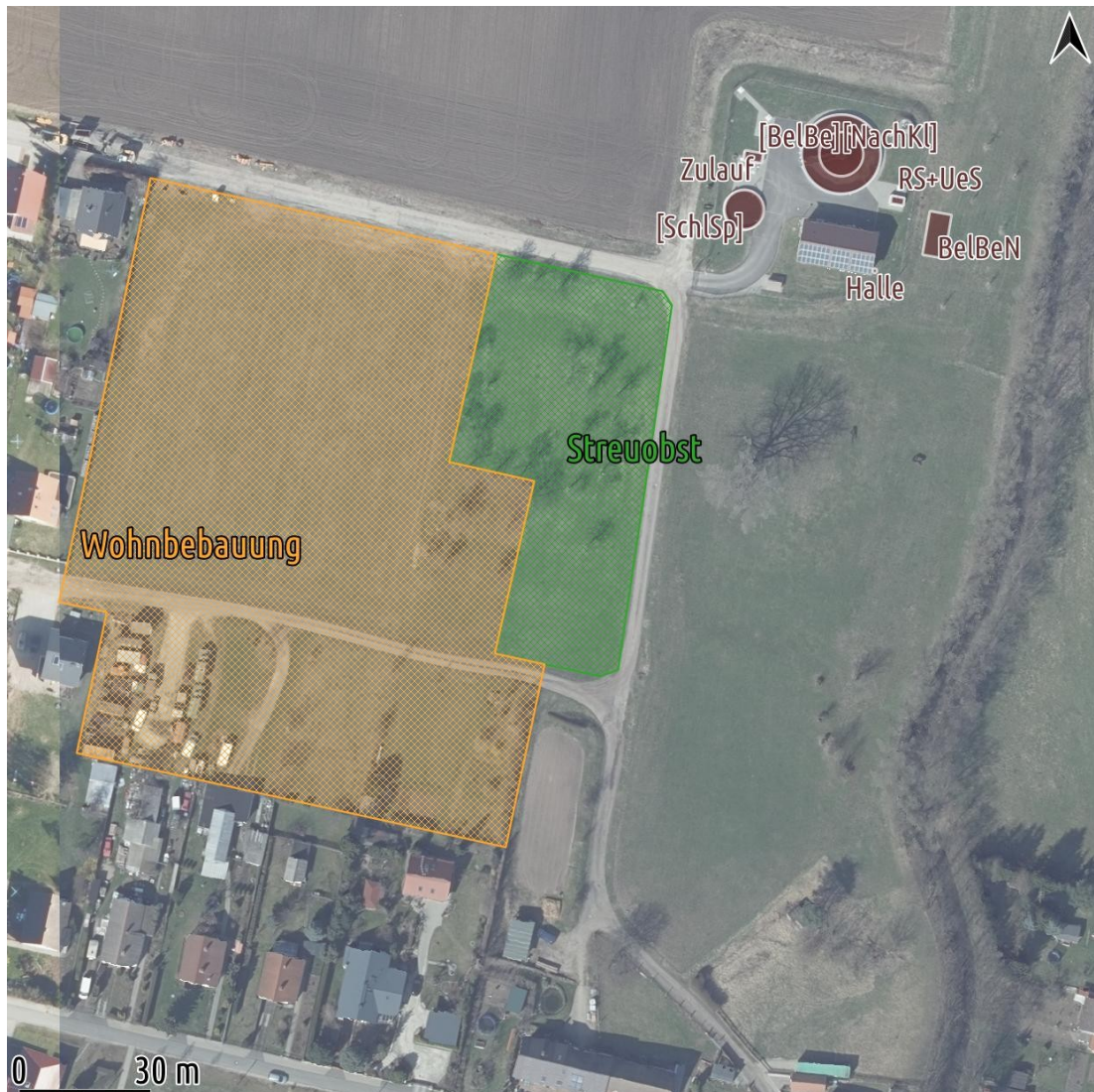
Abb. 1: Lageplan mit den Emissionsquellen der Kläranlage, orthogonale Draufsicht 248 x 248 m 2 von {32641988;5632244} bis {32642236;5632492} | Kartengrundlage: DOP, TLBG
