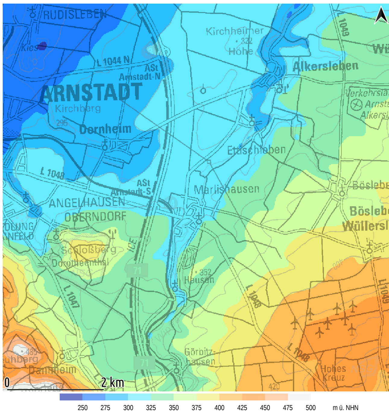
Abb. 4: digitales Höhenmodell DGM200, per Spline-Interpolation übertragen auf eine Maschenweite von 16 m | Kartenhintergrund: DTK100, TLBG
