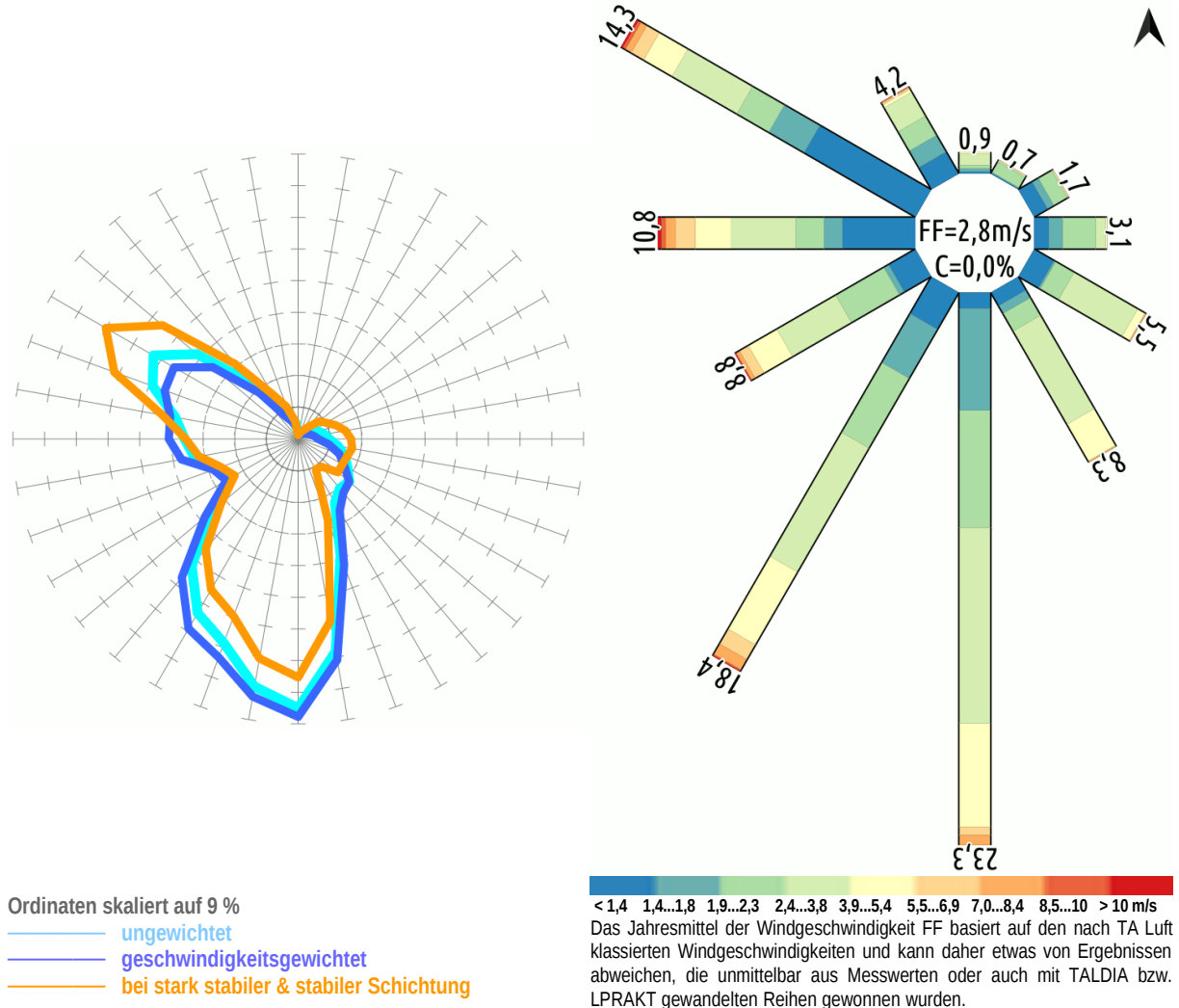
Abb. 12: Häufigkeitsverteilungen der Windrichtung (jeweils normiert auf 100%)
