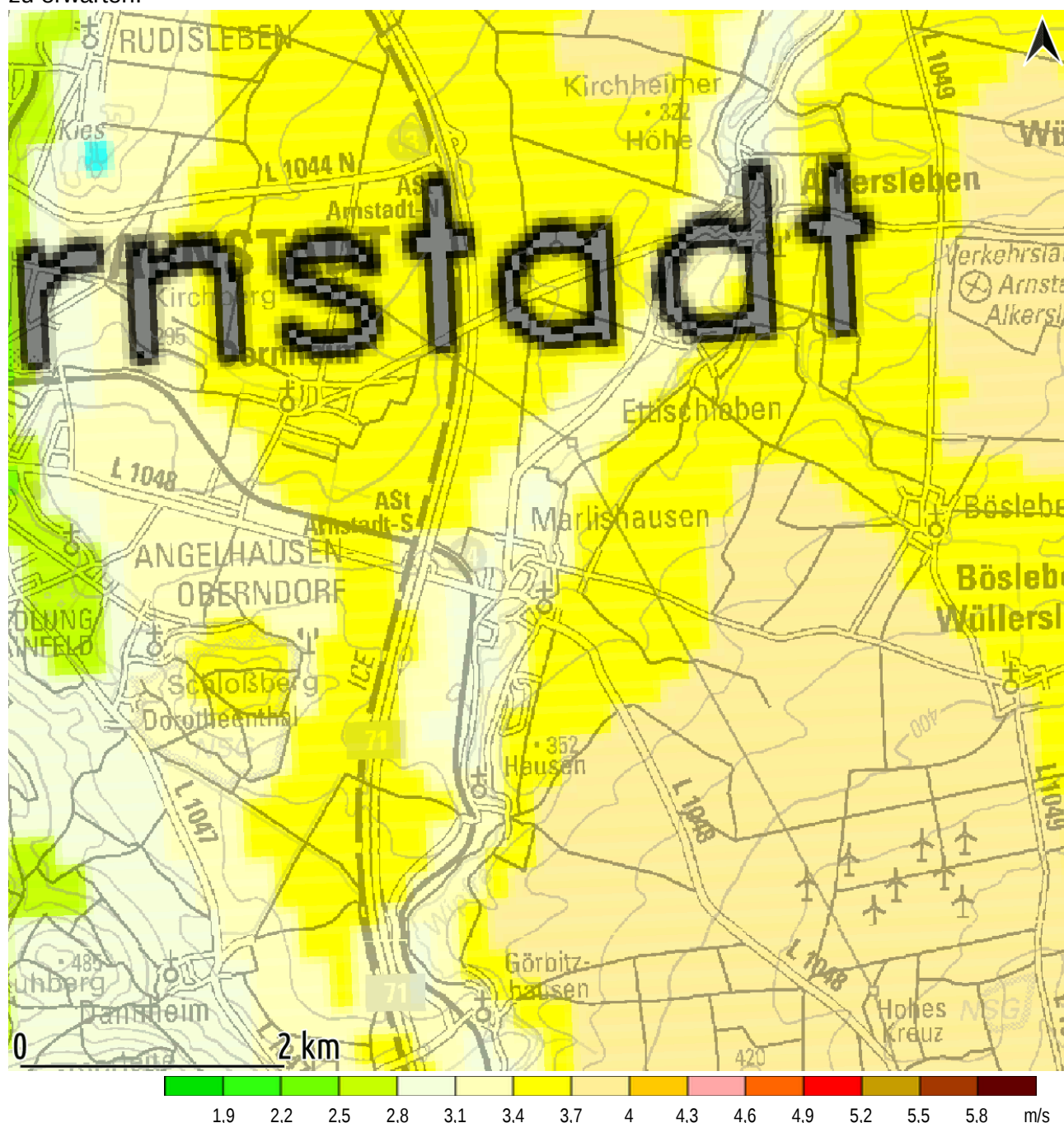
Abb. 7: Windgeschwindigkeitsverteilung nach dem Statistischen Windfeldmodell (SWM) des DWD | Kartenhintergrund: DTK100, TLBG
