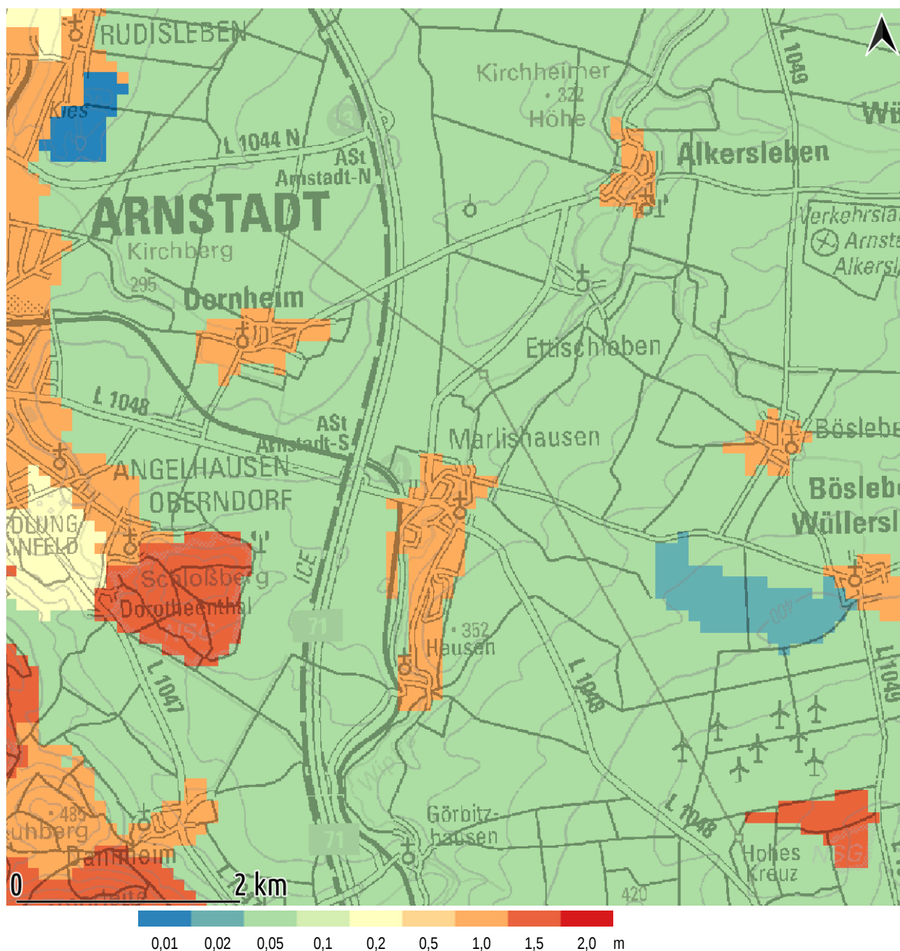
Abb. 6: Rauigkeitslänge z_0 nach CORINE zu AUSTAL2000(N) im UTM-Koordinatensystem, Maschenweite 100 m | Kartenhintergrund: DTK100, TLBG
